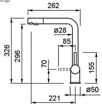
Méreterajz
