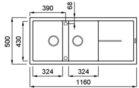
Méretrajz
