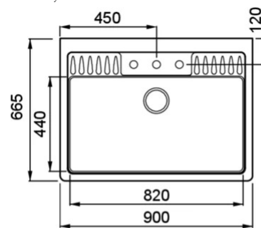
Méretrajz
