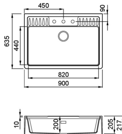
Méretrajz
